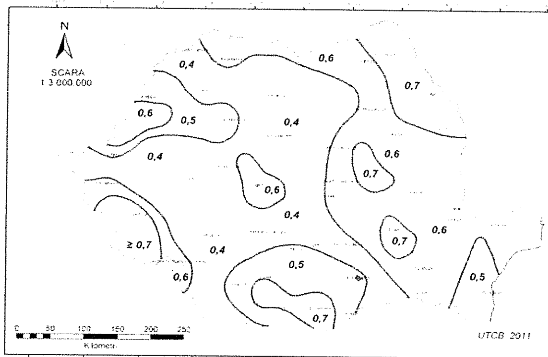
Zonarea valorii caracteristice a încărcării din zăpadă S_{0,k} kN/m
