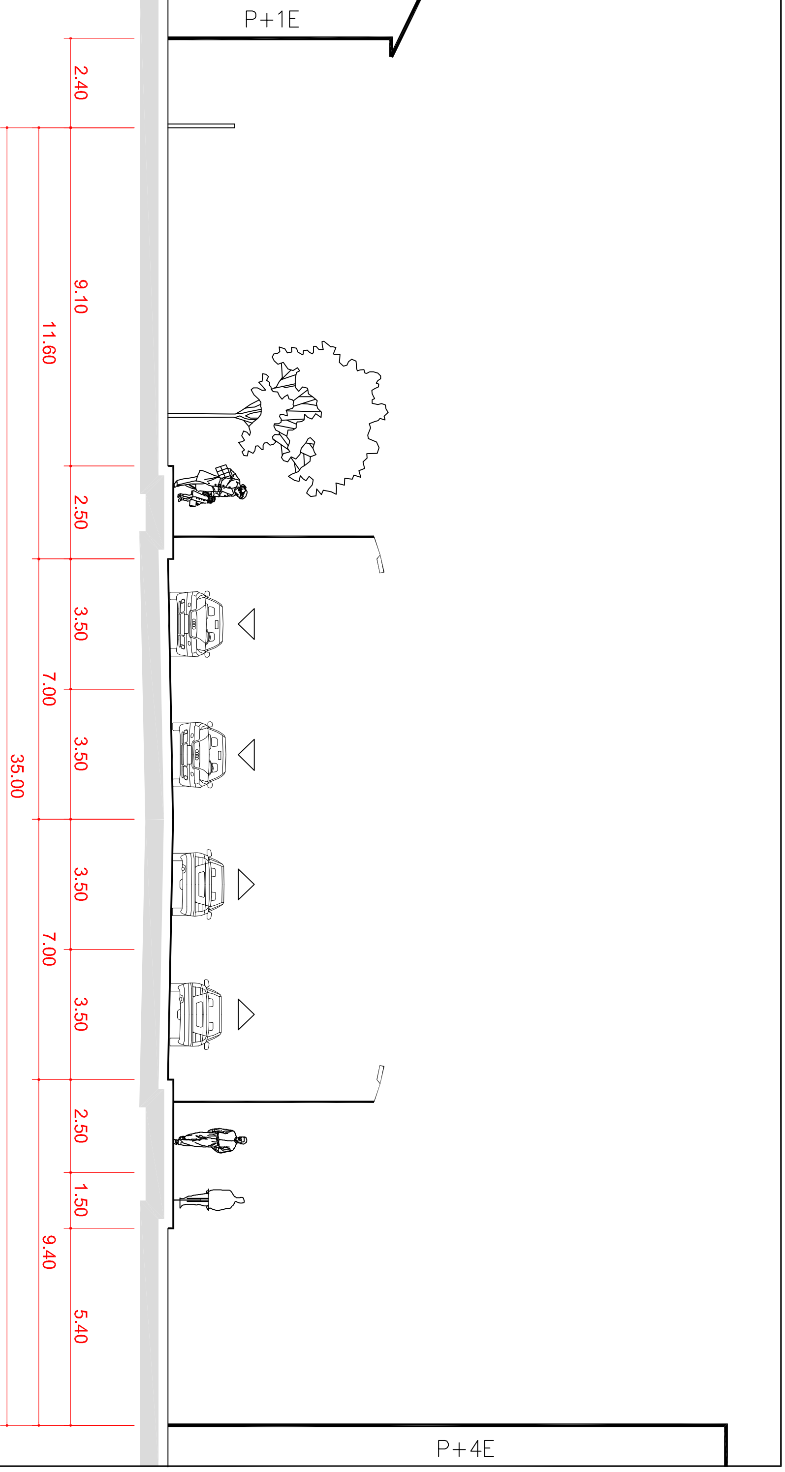
PROFIL D-D
